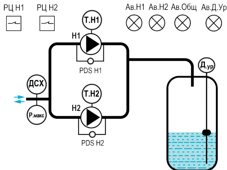
Рисунок 1.7 – Объект управления
